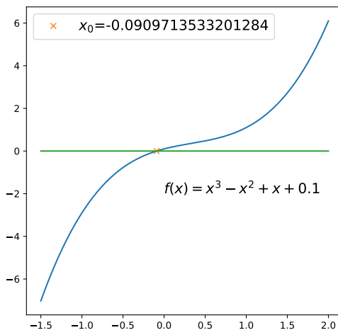
FIGURE 3.1 – Tracé de la fonction f(x) = x^3 - x^2 + x + 0.1 et le point racine obtenu par la méthode de dichotomie en utilisant la bibliothèque scipy
