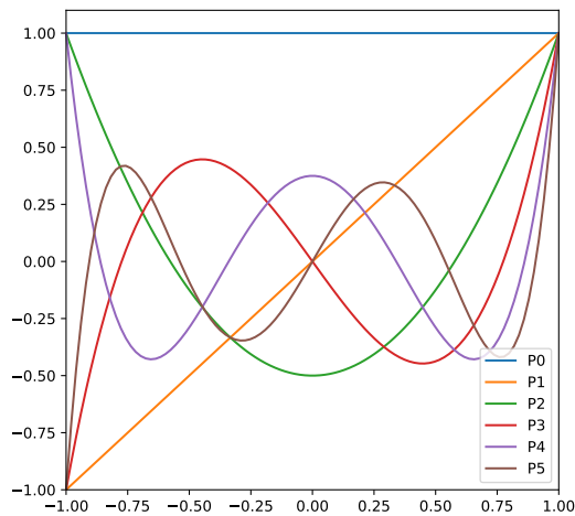
FIGURE 1.2 – Polynômes de Legendre.
