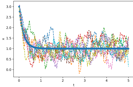
FIGURE 6.3 – 10 trajectoires correspondant au processus d'Ornstein-Uehlenbeck ainsi que la solution exacte pour la valeur moyenne
