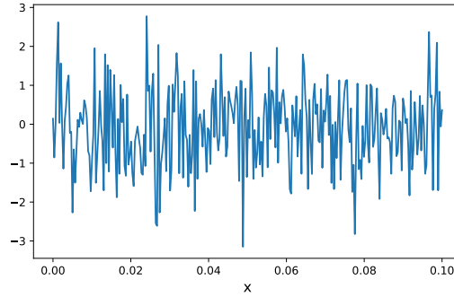
FIGURE 6.2 – Bruit Gaussien à une dimension en fonction du temps
