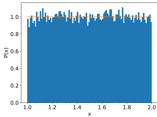
FIGURE 4.2 – Comparaison d'un histogramme de nombres aléatoires d'une distribution uniforme et de la probabilité d'un nombre infini de tirages.
