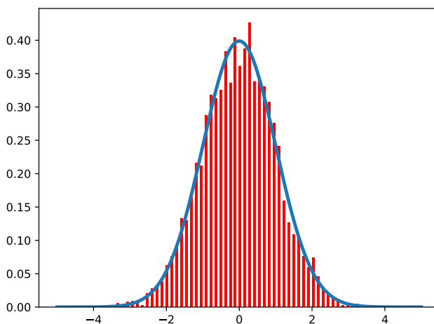
FIGURE 4.3 – Comparaison d'un histogramme de nombres aléatoires d'une distribution gaussienne et de la probabilité d'un nombre infini de tirages.
