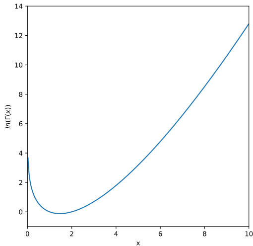
FIGURE 7.2 – Fonction lngamma
