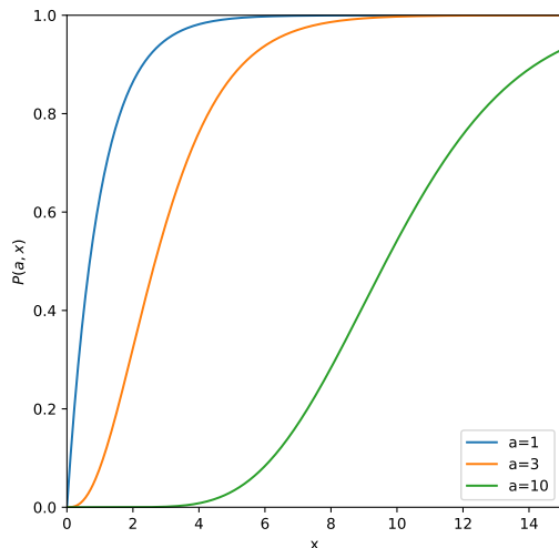
FIGURE 7.3 – Fpncions gamma incomplètes On définit la fonction \gamma incomplète comme
