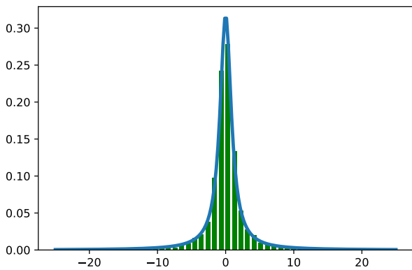
FIGURE 4.4 – Comparaison d'un histogramme de nombres aléatoires d'une distribution de Cauchy centrée sur l'origine et de la probabilité d'un nombre infini de tirages.
